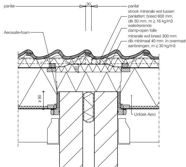
Detailtekening 1 - Woningsecheidende wand Unidek Aero
