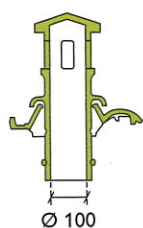
doorvoerpan (met doorvoer voor dakhelling 25° - 45°)
