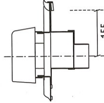
universele Combipan® (geometrische doorlaat 12.200 mm 2 )
